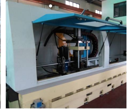
High Speed 2-Knife Cutter (Motion Control) 高速雙刀式切管機
